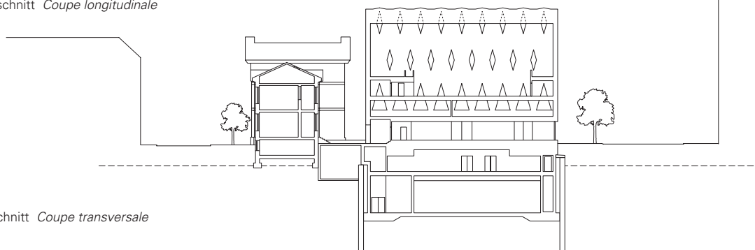
Längsschnitt Coupe longitudinale
