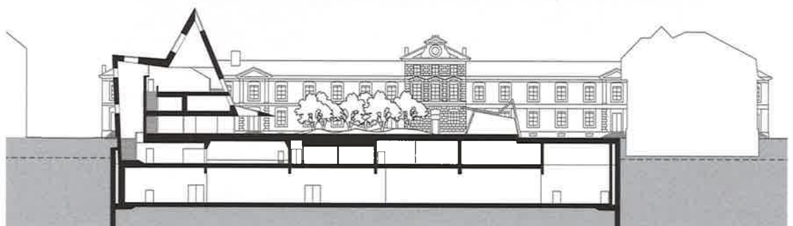
Längsschnitt
