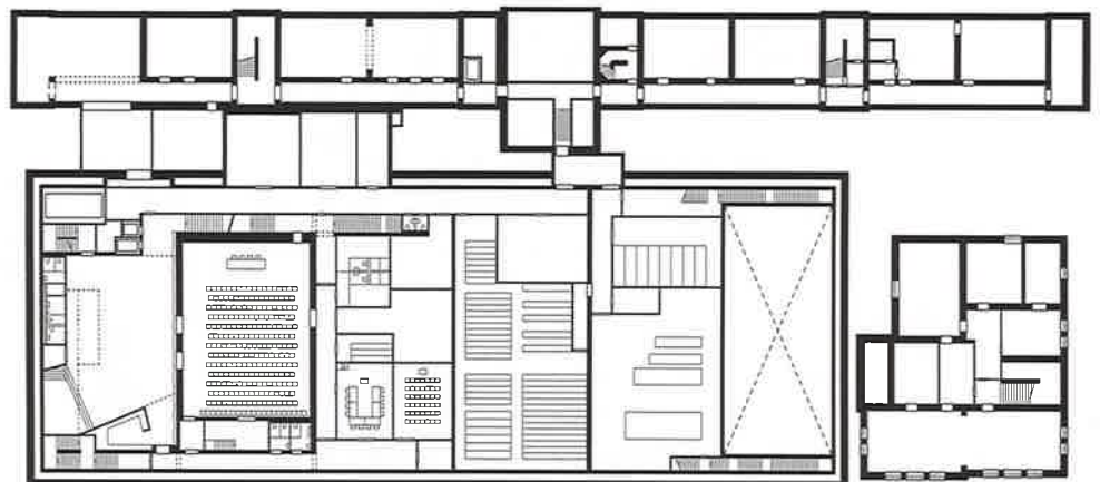
1. Untergeschoss
