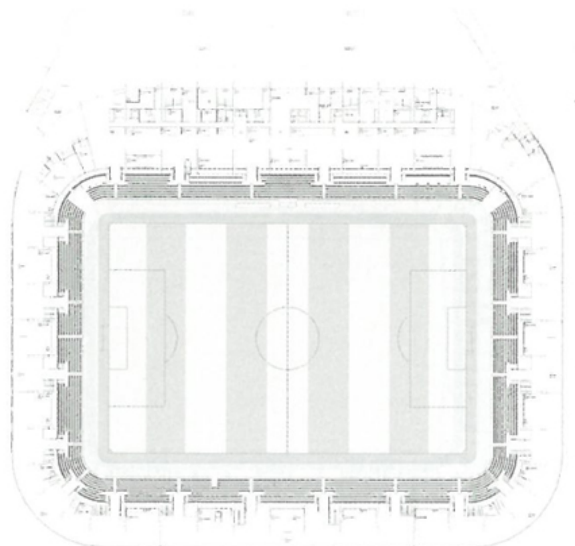
OG 1 M 1:2.000 Verteilerebene und Stadionmanagement
