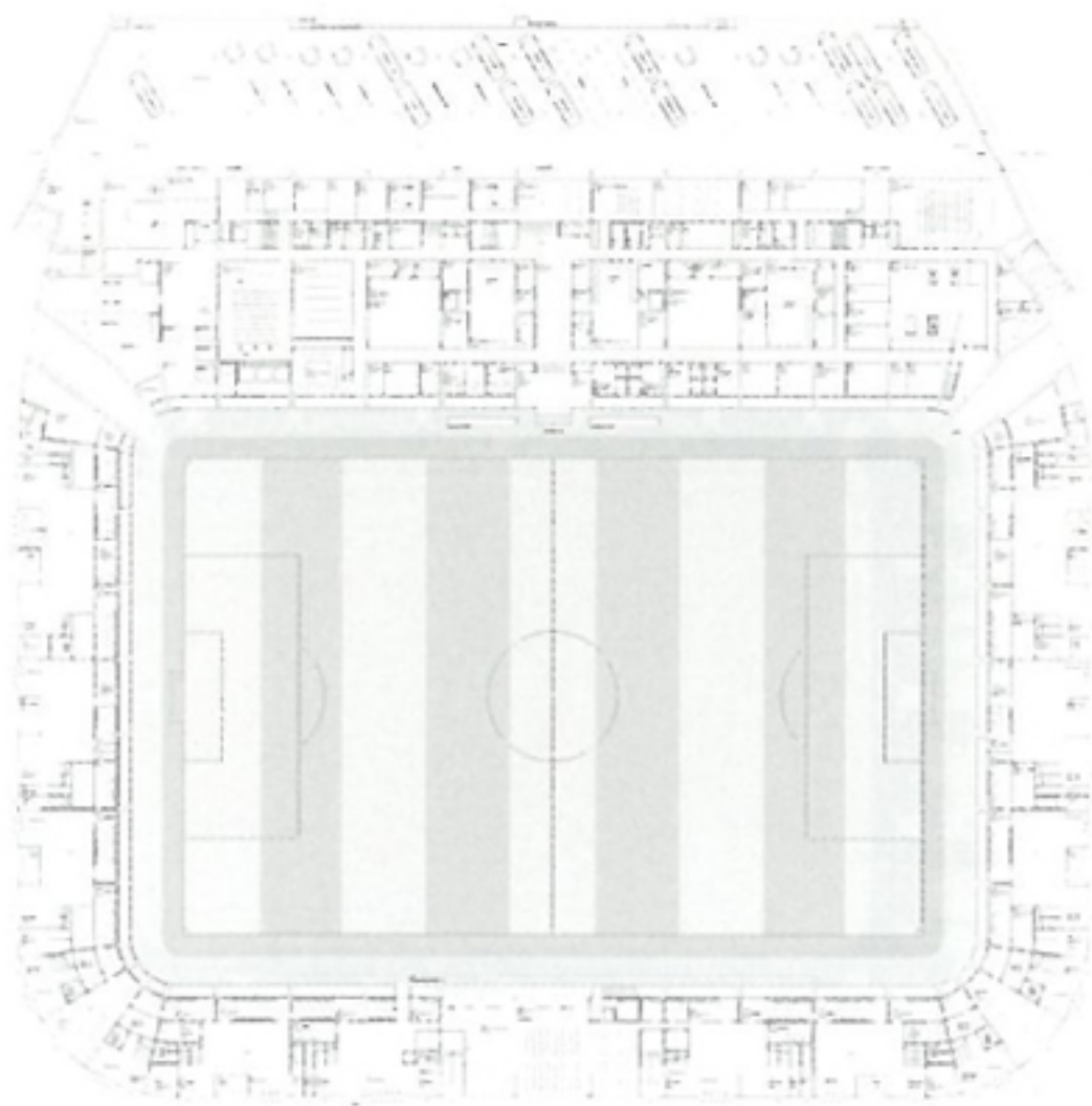
EG M 1:2.000 Spielbetrieb, Medien und Gastronomie
