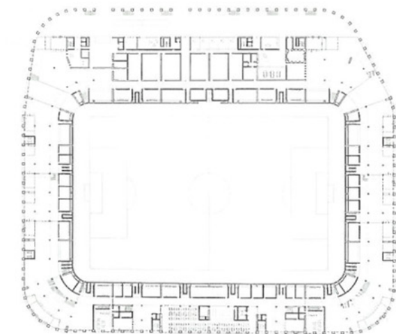
Grundriss EG M 1:2.000
