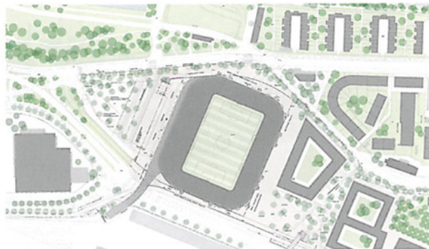
Lageplan M 15 000
