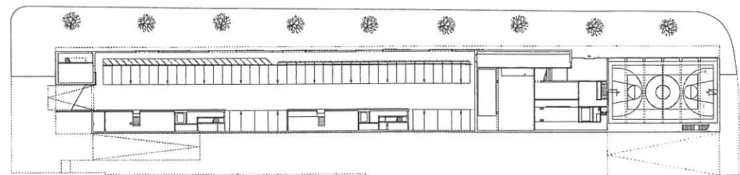
Sockelgeschoss mit Parkgarage und Turnhalle
