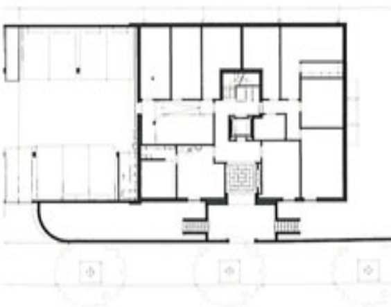
^ Eingangsgeschoss Kollhoff
